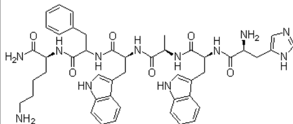
His-D-Trp-Ala-Trp-D-Phe-Lys-NH 2
